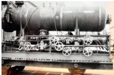
Abscheider(II) für das Erdgasförderfeld Salzwedel/Peckensen aus dem Leistungsspektrum des Stahlbaus im ZRAW Zeitzeugen-Archiv
